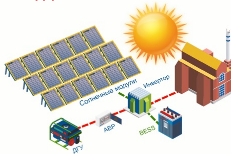
Установка дизель гибридной СЭС
