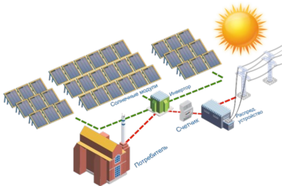
Установка On-Grid систем для планируемых объектов
